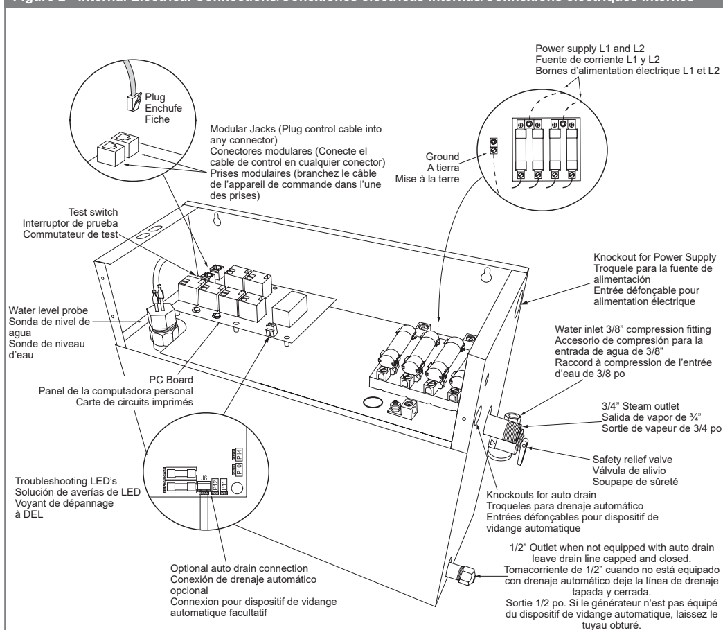
Figure 2 - Internal Electrical Connections/Conexiones eléctricas internas/Connexions électriques internes
