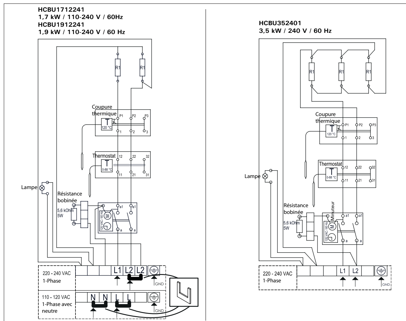
Figure 6. Connexions électriques de poêle
